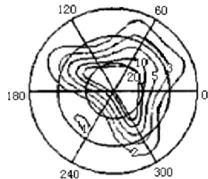
图 4 液晶的视角特性
