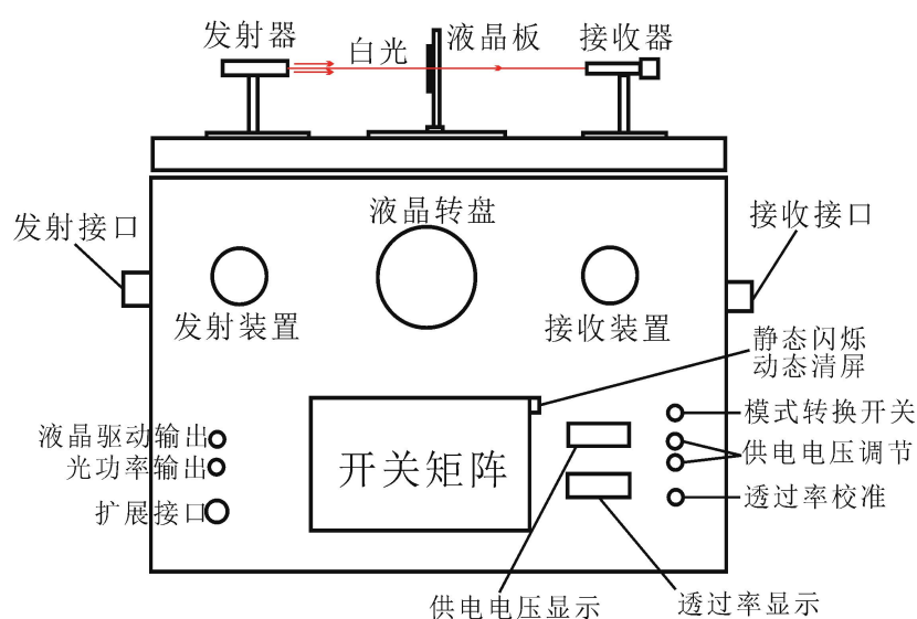
图 6 液晶光开关电光特性综合实验仪功能键示意图
