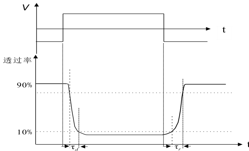
图 3 液晶驱动电压和时间响应图
