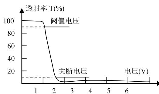
图2 液晶光开关的电光特性曲线
